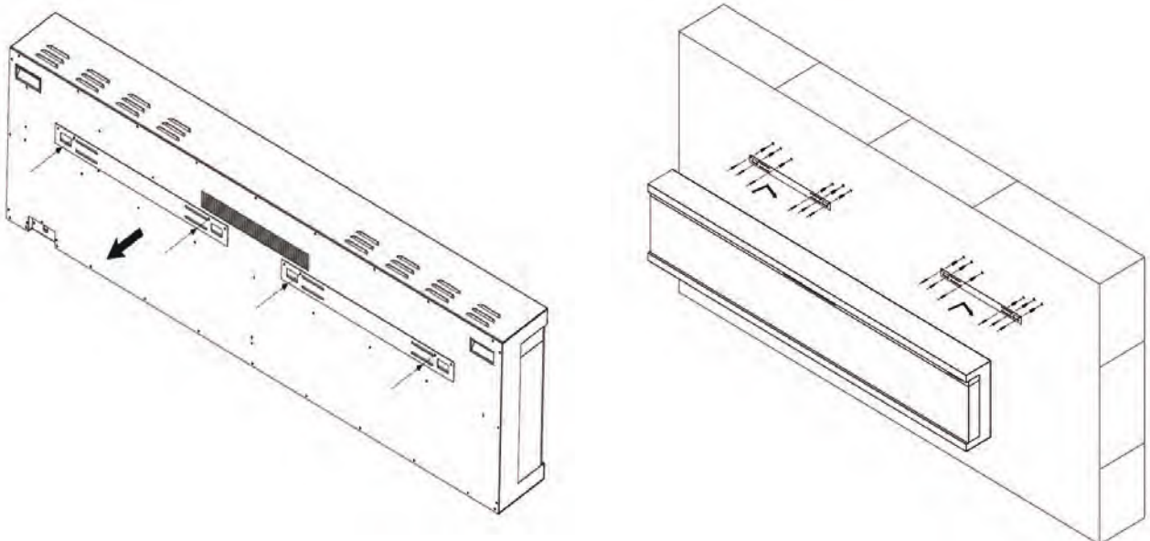
Abbildung der Wandhalterung für Modell EF-U183
