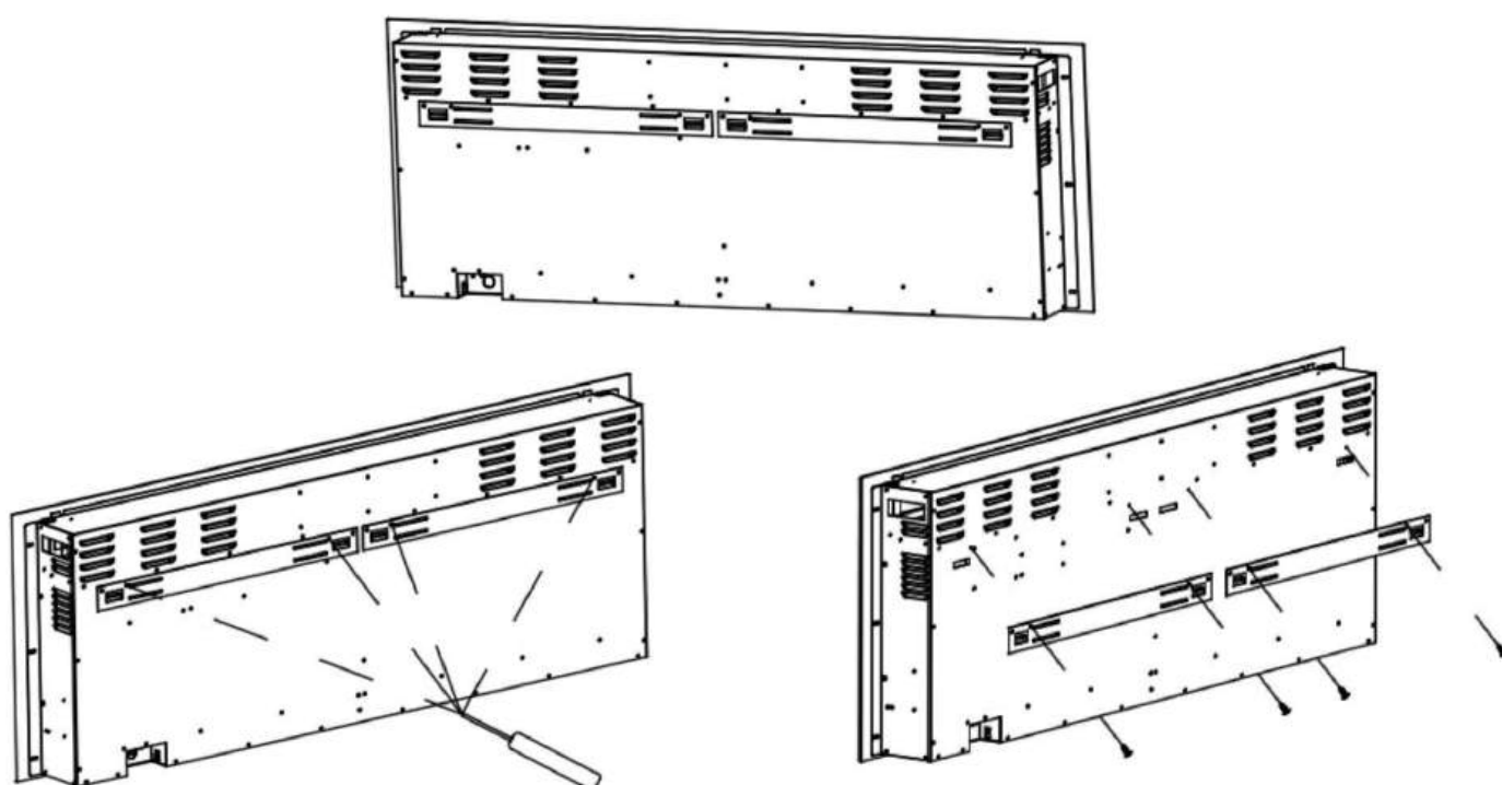
Illustration du support mural pour les modèles 254
