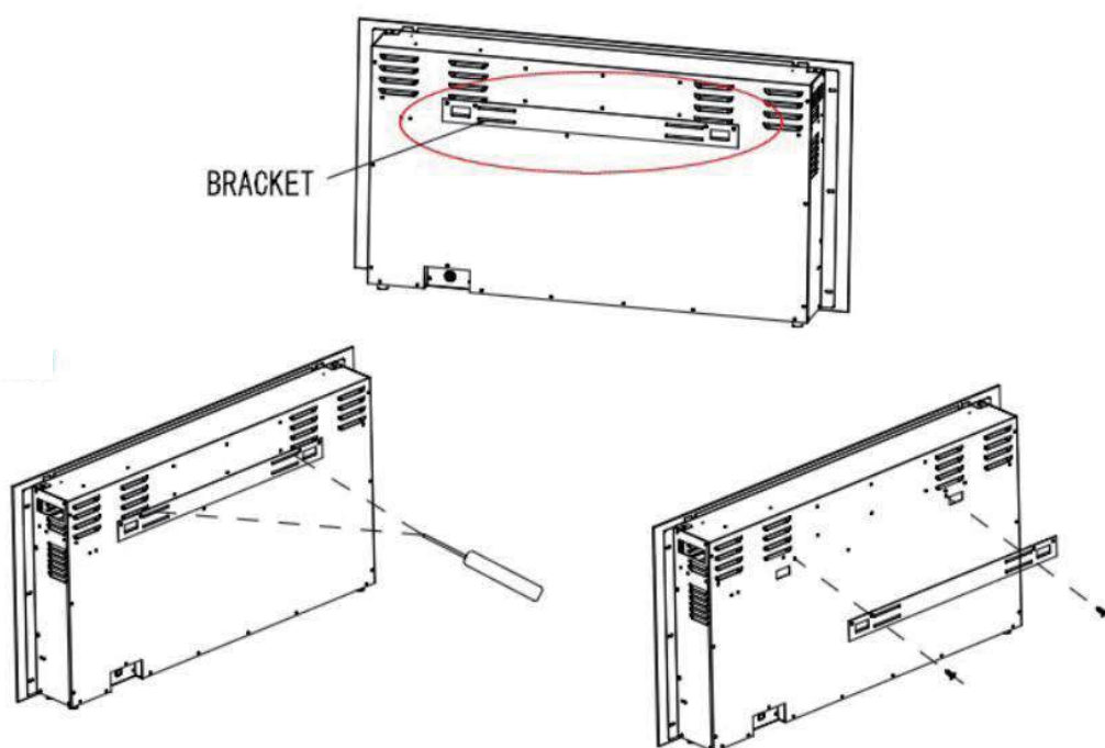
Illustration du support mural pour les modèles 107/128/153/183/213
